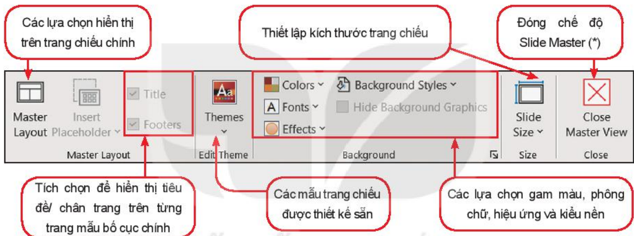
Hình 1.3. Các lệnh định dạng trang chiếu chính trong chế độ Slide Master
