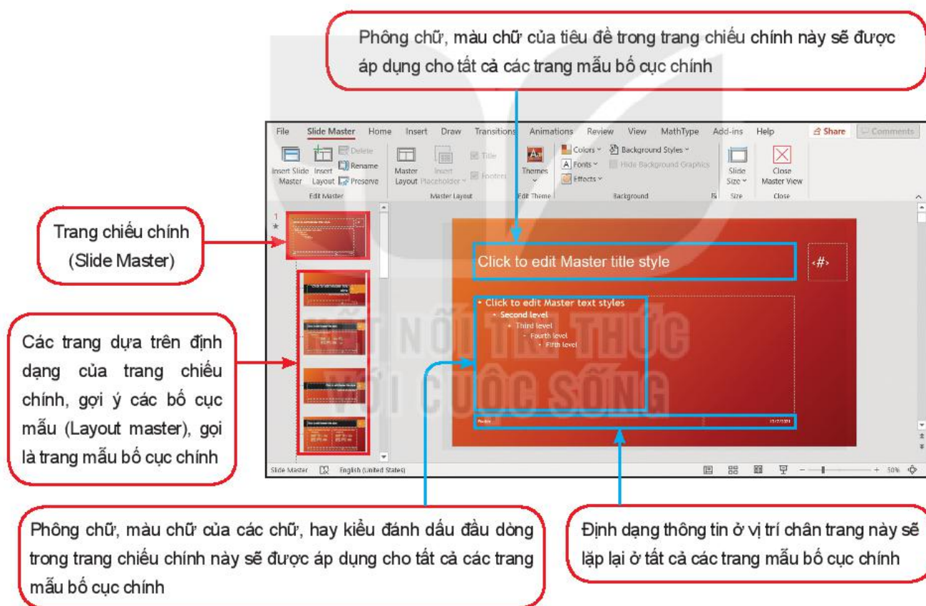
Hình 1.2. Màn hình soạn thảo ở chế độ Slide Master
