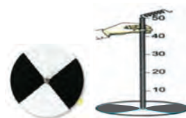
Hình 13.8. Cấu tạo đĩa Secchi
