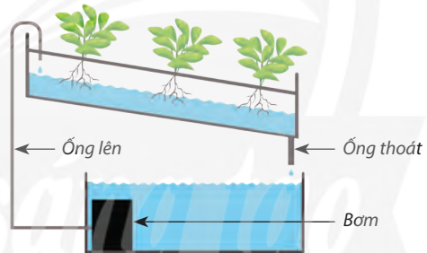
Hình 2.5. Hệ thống thủy canh hồi lưu
