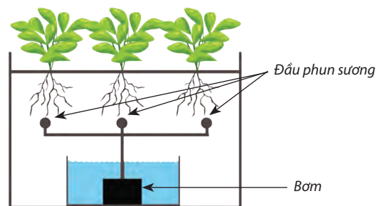
Hình 2.6. Hệ thống khí canh
