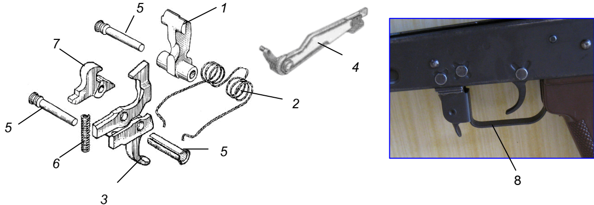
Hình 4-10. Bộ phận cò
