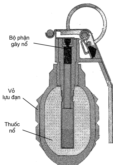
Hình 6-4. Cấu tạo lựu đạn cân 97
