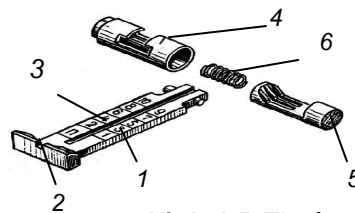
Hình 4-5. Thước ngắm
