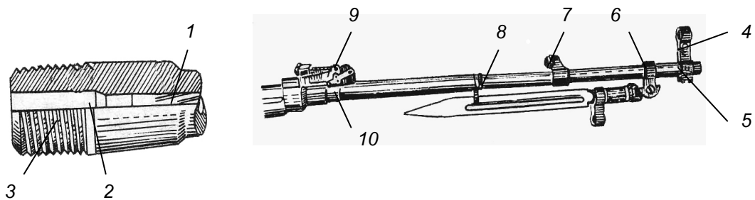
Hình 4-31. Nòng súng
