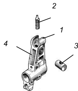
Hình 4-4. Đầu ngắm
