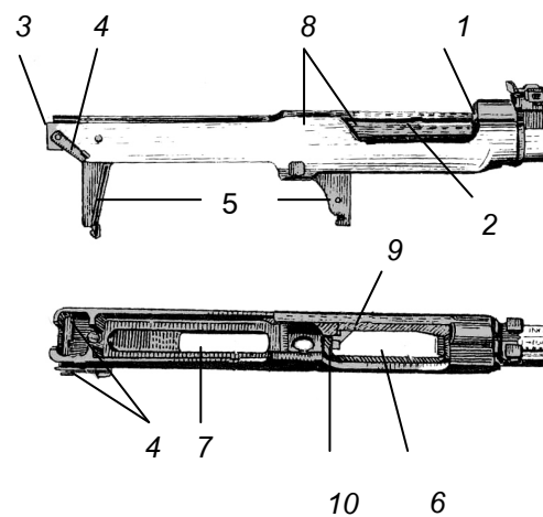
Hình 4-34. Hộp khoá nòng
