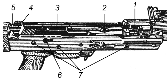
Hình 4-6. Hộp khoá nòng
