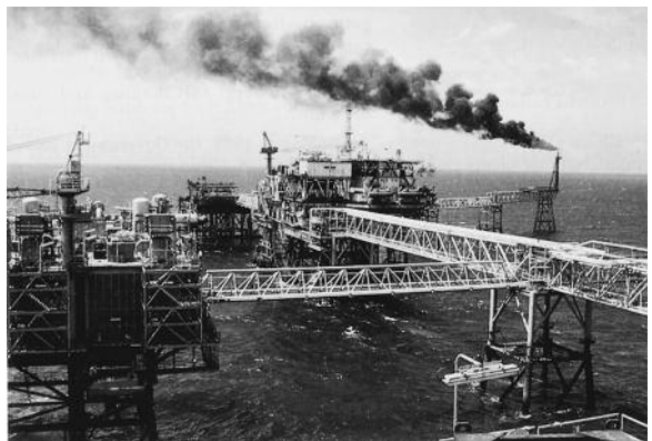
Hình 88. Khai thác dầu ở mỏ Bạch Hổ trên Biển Đông
