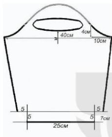
Bản vẽ thông số kích thước
