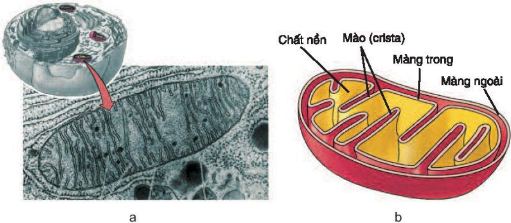
Hình 9.1. Cấu trúc của ti thể a) Ảnh chụp lát cắt ngang của ti thể dưới kính hiển vi điện tử; b) Sơ đồ cấu tạo của ti thể.
