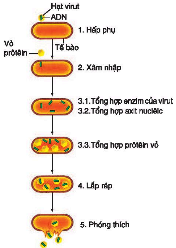
Hình 30. Chu trình nhân lên của phagơ
