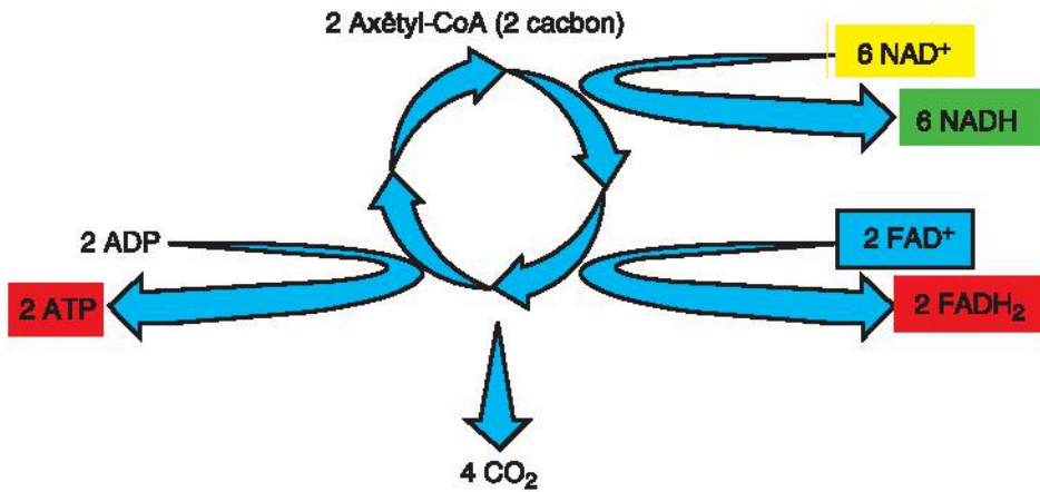
Hình 16.3. Sơ đồ tóm tắt chu trình Crep
