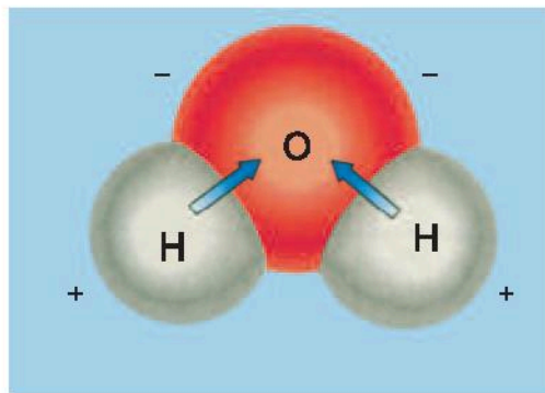
Hình 3.1. Cấu trúc của phân tử nước
