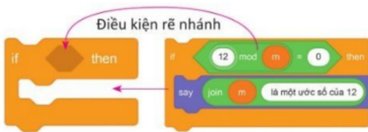
Hình 2a. Khối lệnh để thể hiện rẽ nhánh khuyết
